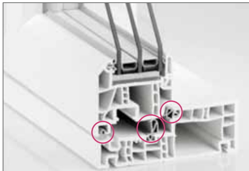
Tre omløbende tætningsniveauer
